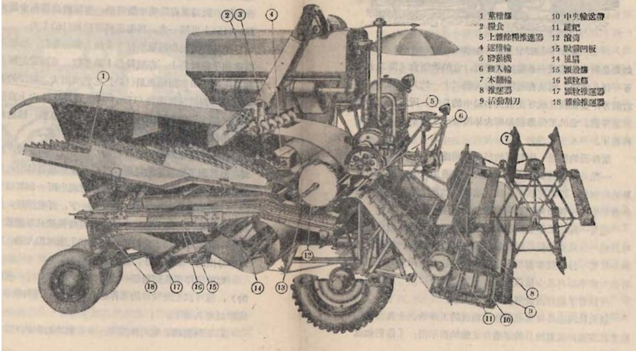
圖二十 斯大林涅茨-4(C-4)自動聯合收割機結構圖
